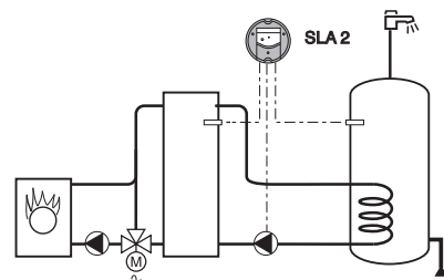
RÉGULATION DIFFÉRENTIELLE SLA 2 - COLIS EC320
